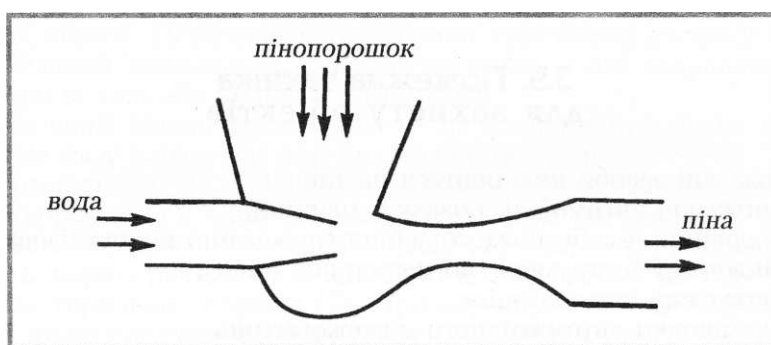
Рис. 12. Схема піногенератора
