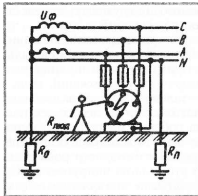
Рис. 26. Занулення
