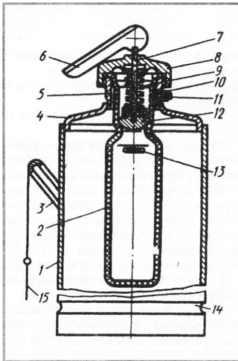
Рис. 13. Вогнегасник ВХП-10: 1 — корпус; 2 — кислотний стакан; 3 — бокова ручка; 4 — перехідник; 5 — горловина; 6 — рукоятка; 7 — шток; 8 — кришка; 9 — пружина; 10 — сприск; 11 — мембрана; 12 — гумовий клапан; 13 — рівень кислотної частини; 14 — дно; 15 — голка
